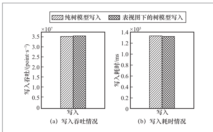
图12 是否使用表视图对写入性能的影响分析
