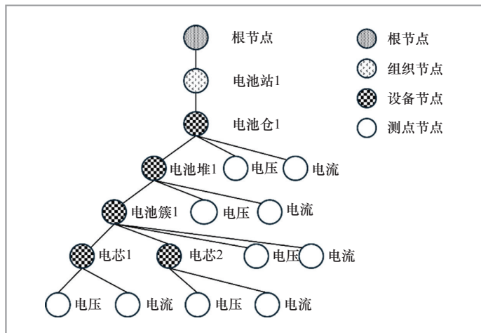
图4 树模型示例
